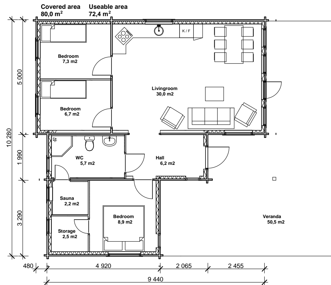
2. Plan 1:100
