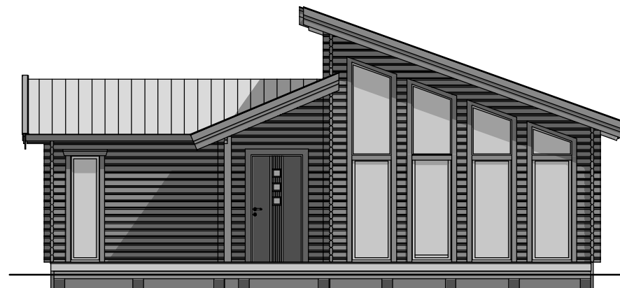
A2 Elevation 1:100
