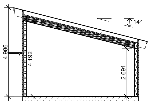
S3 1:100
