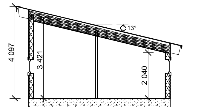
S1 1:100
