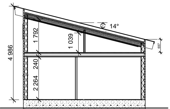
S2 1:100
