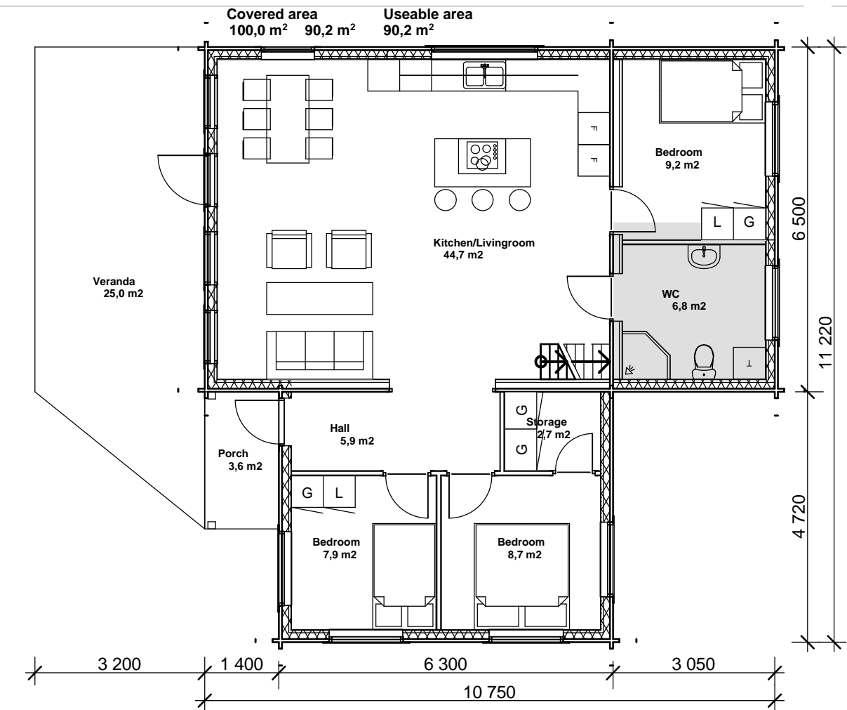
2. Plan 1:100
