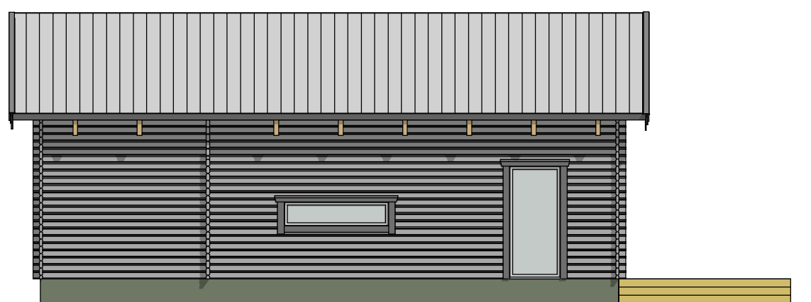
A3 Elevation 1:100
